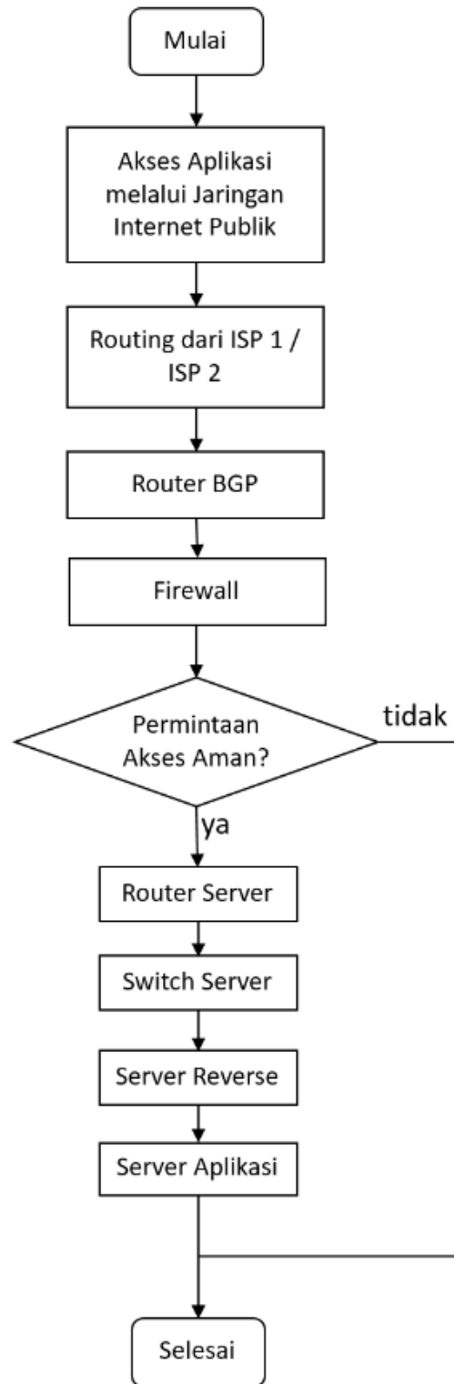
Gambar 5. Alur akses data dari Internet Publik ke server Aplikasi Pemerintah Kota Madiun
